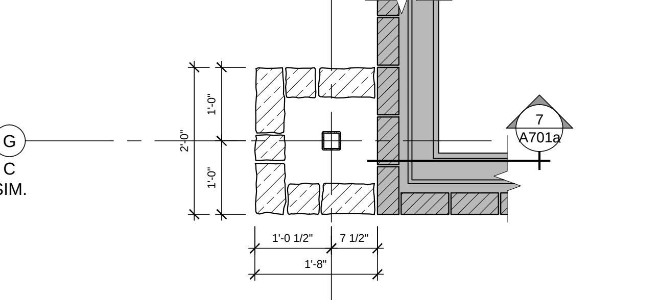
PIERS C3, D3, E3 & F3 - FOUNDATION PLAN
