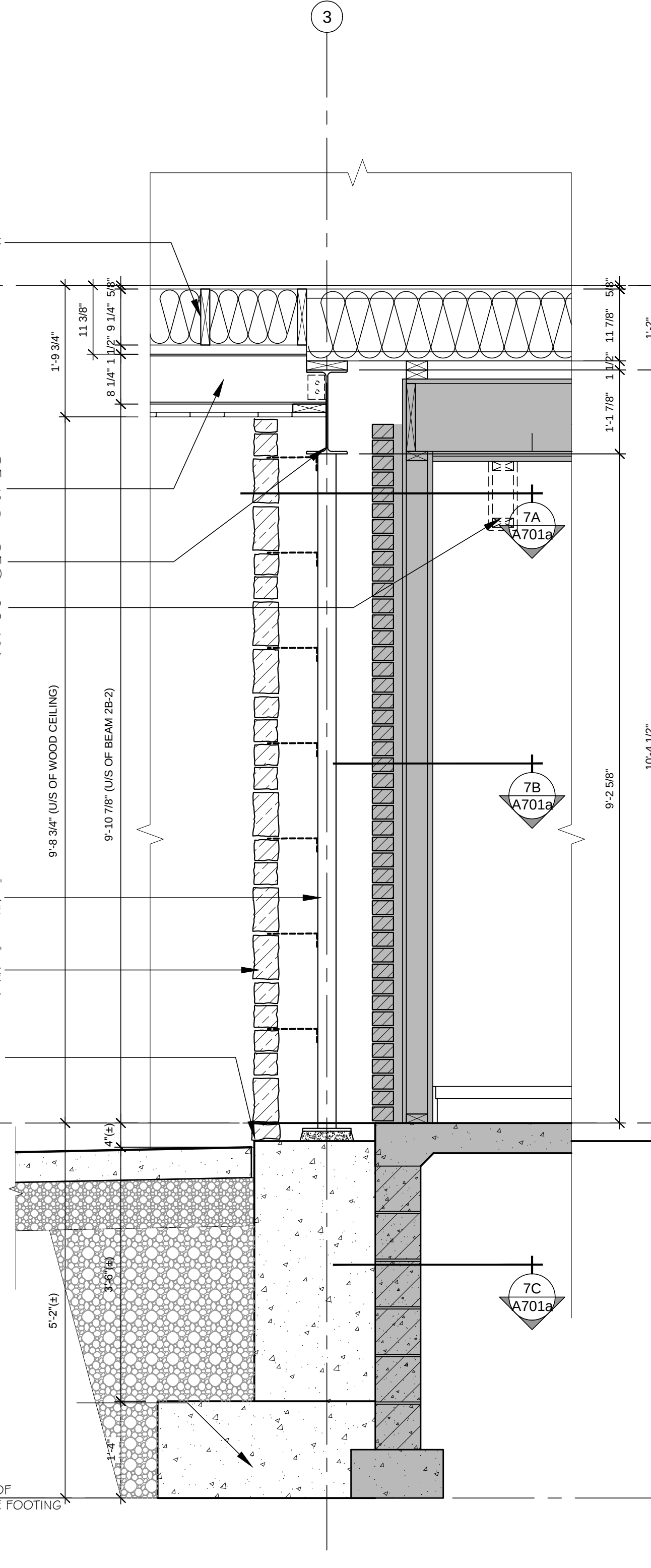
PIER C3, D3, E3 & F3 - SECTION
