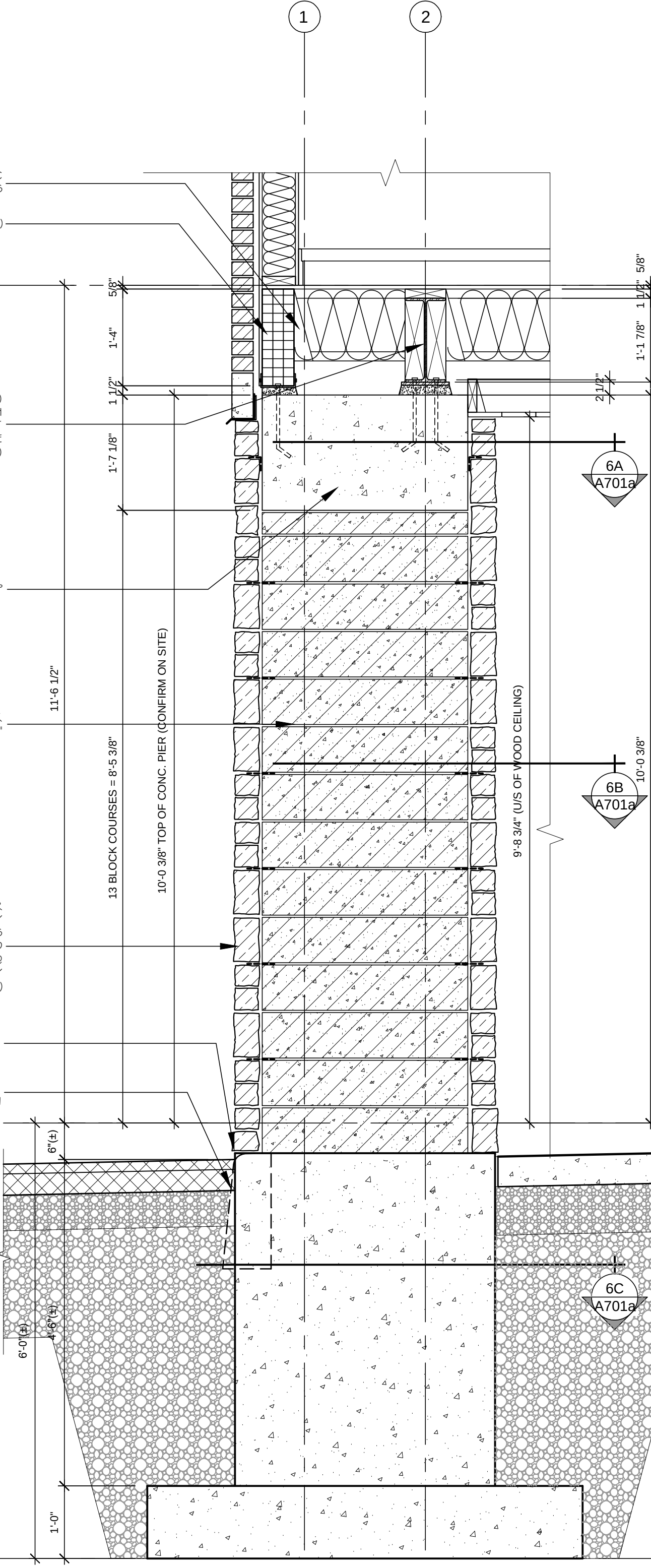
PIER D1.2, PIER F1.2 (SIM) - SECTION
