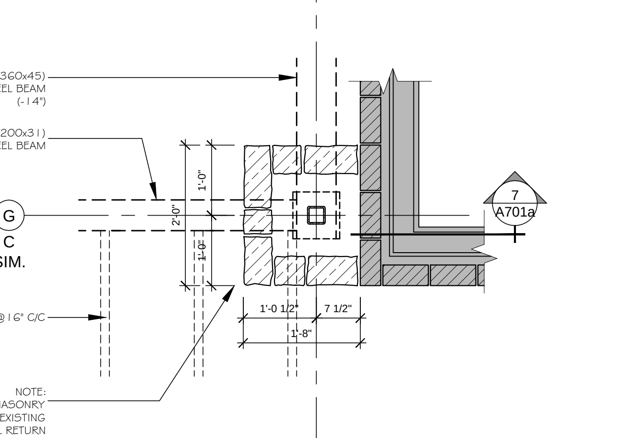
PIER C3, D3, E3 & F3 - UPPER PLAN
