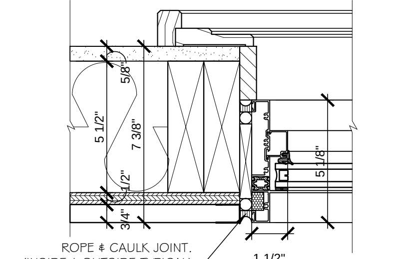
WINDOW JAMB (TYP) SCALE: 3"=1'-0"
