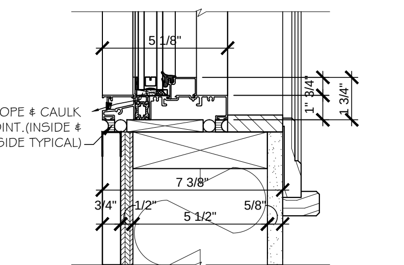
WINDOW SILL (TYP) SCALE: 3"=1'-0"
