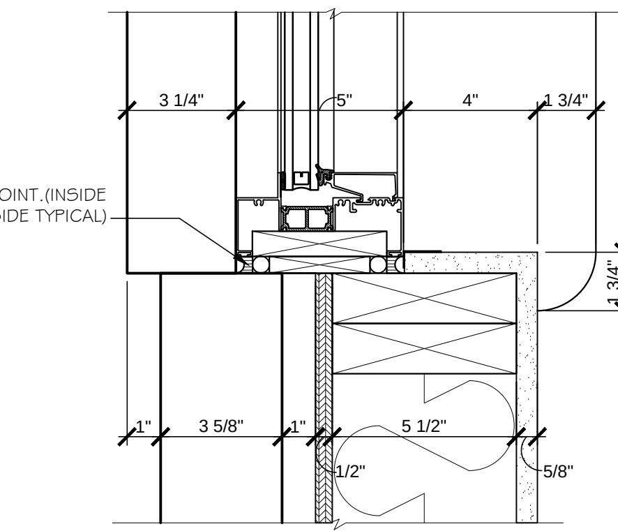
WINDOW JAMB (TYP) SCALE: 3"=1'-0"
