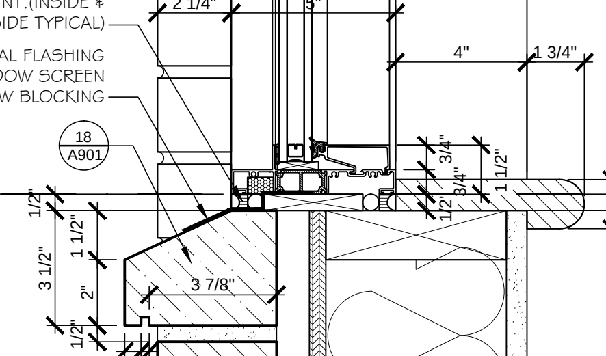
WINDOW SILL (TYP) SCALE: 3"=1'-0"
